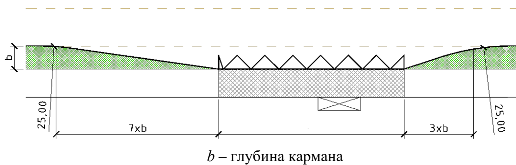
Рисунок В.1 – Остановочный пункт с параллельным карманом
